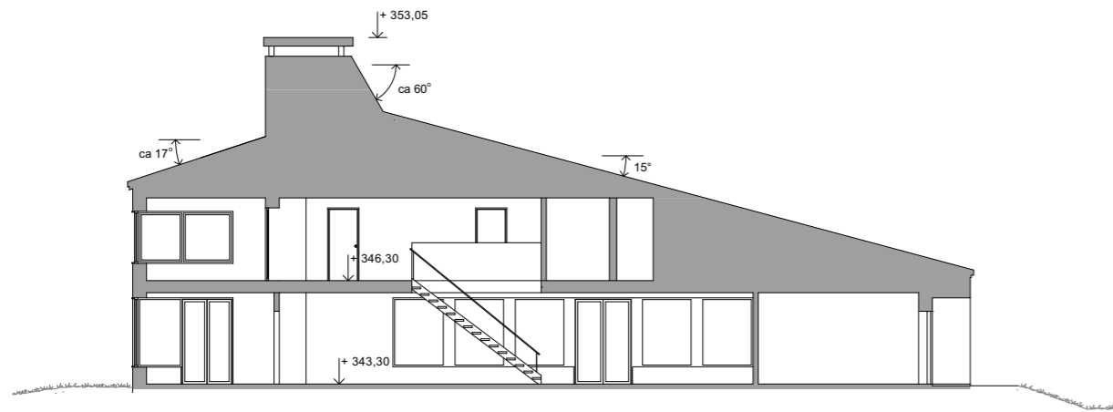
sektion
