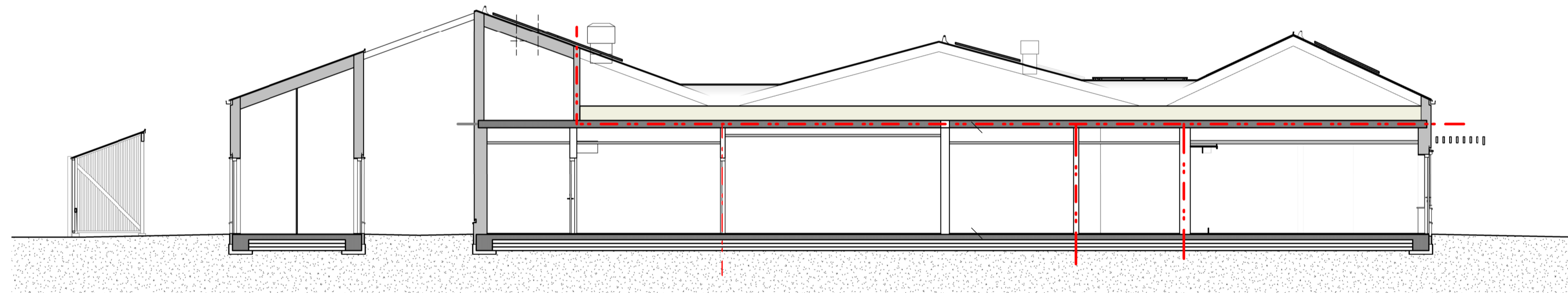
SEKTION B-B
