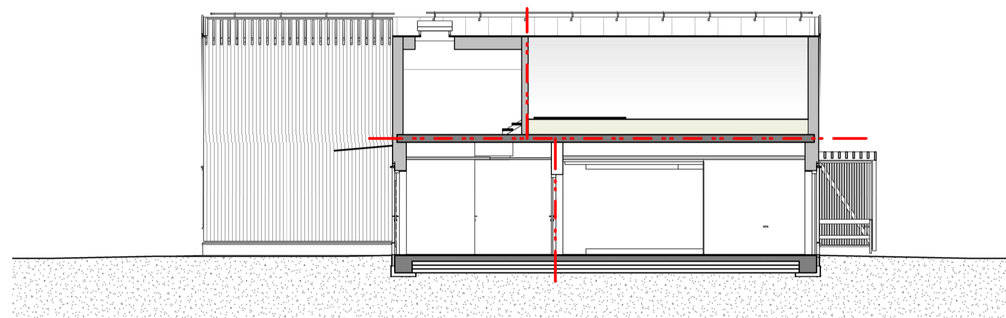
SEKTION E-E
