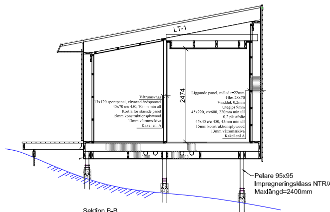
Sektion B-B
