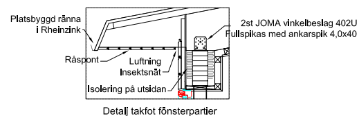
Detalj takfot fönsterpartier
