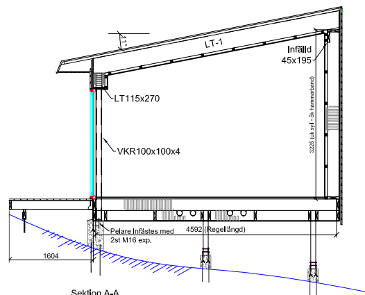
Sektion A-A
