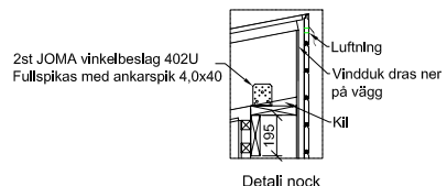
Detaljnock
