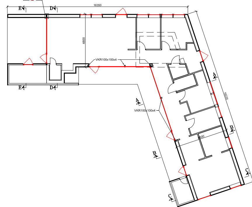
Detalj stomme
