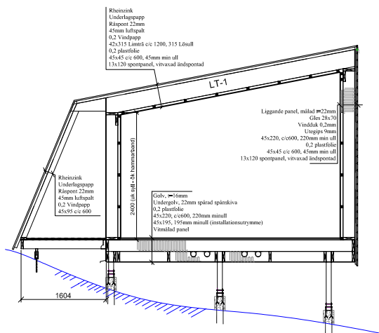
Sektion C-C
