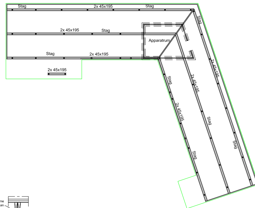
Detalj stomme
