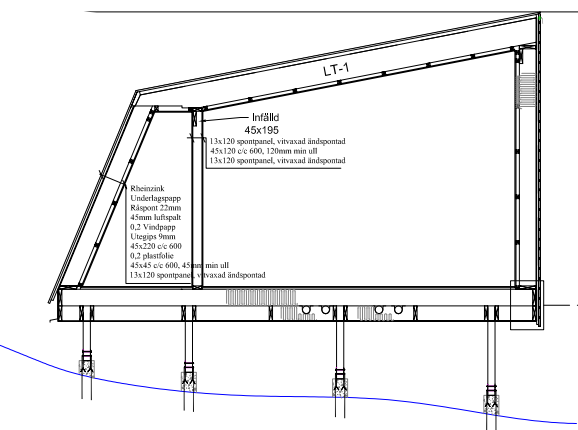
Sektion D-D
